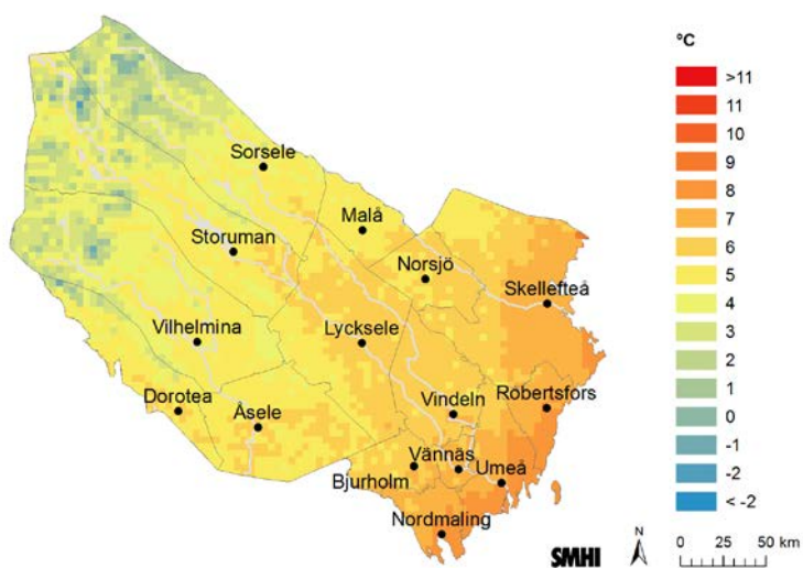
Scenario RCP 8.5
